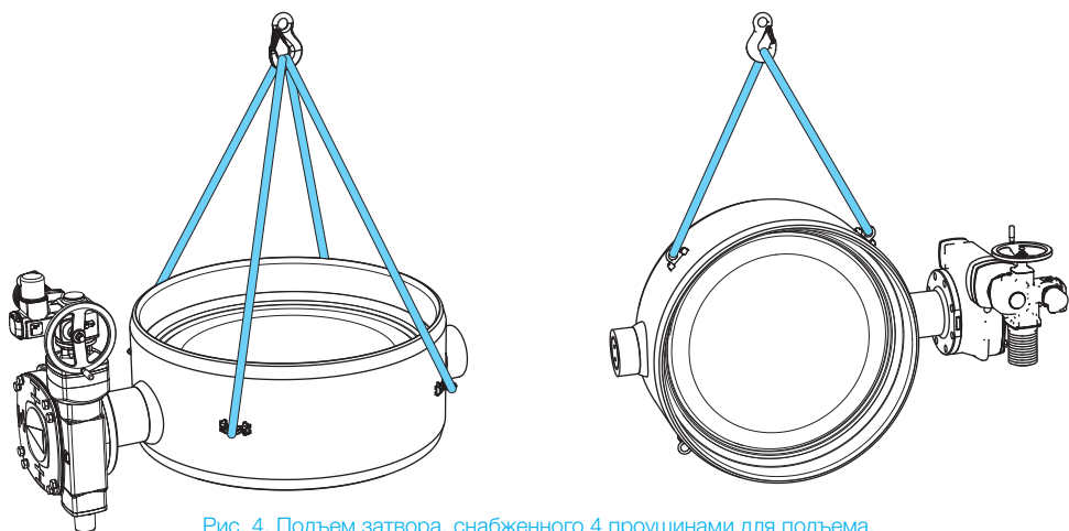
Рис. 4. Подъем затвора, снабженного 4 проушинами для подъема.
