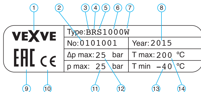
Рисунок 1. Заводская табличка.
